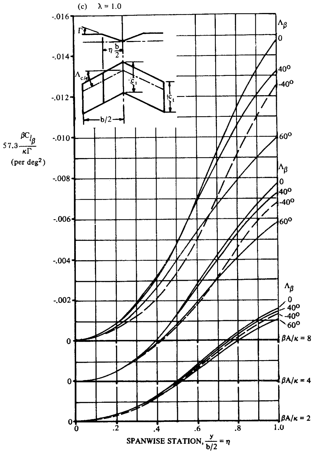
FIGURE 5.1.2.1-31 (CONTD)
