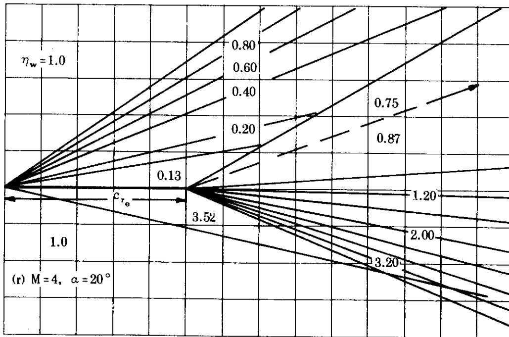
FIGURE 5.6.1.2-9 TAIL EFFECTIVENESS PARAMETER (contd)
