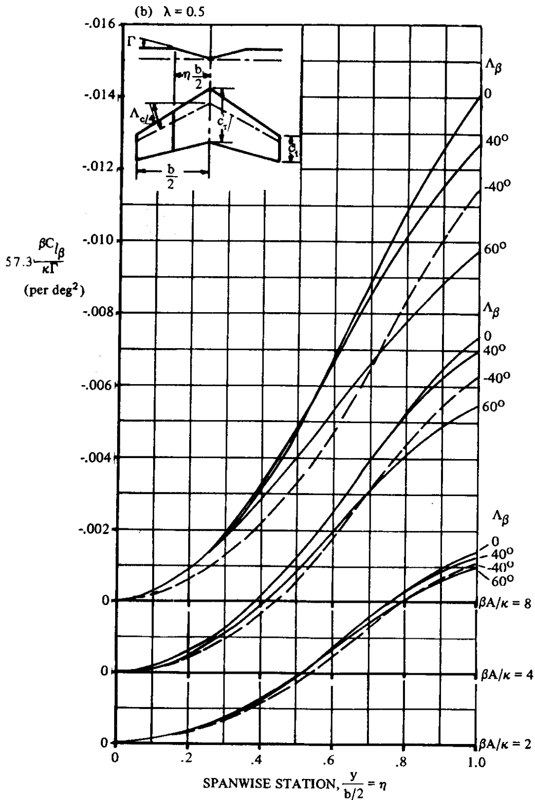
FIGURE 5.1.2.1 -31 (CONTD)
