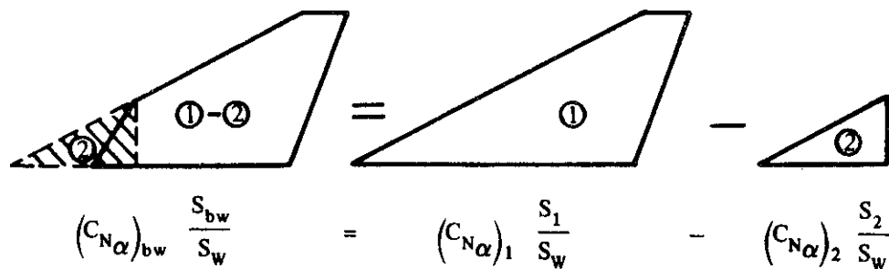
SKETCH (d)
